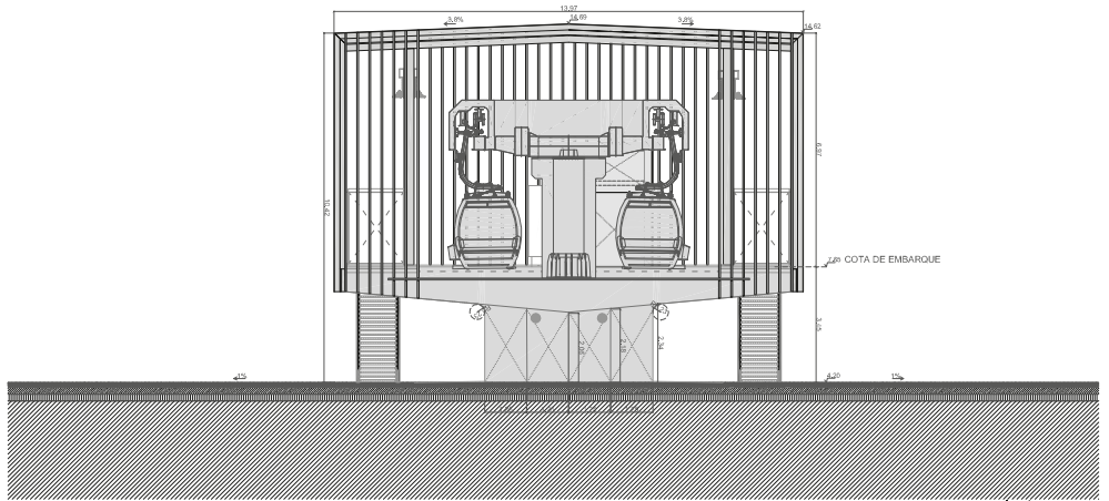
alçado nascente
