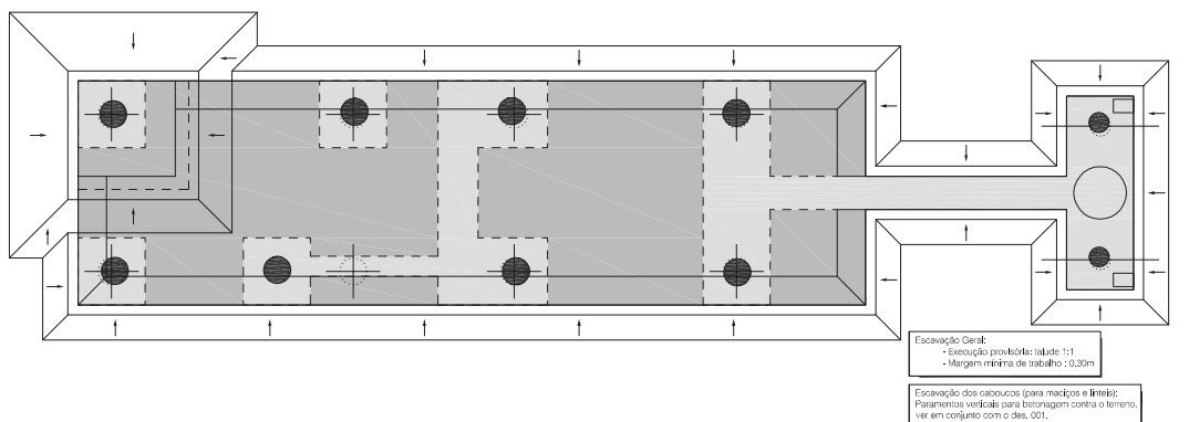
planta - zona de abertura de cabouços para fundações
