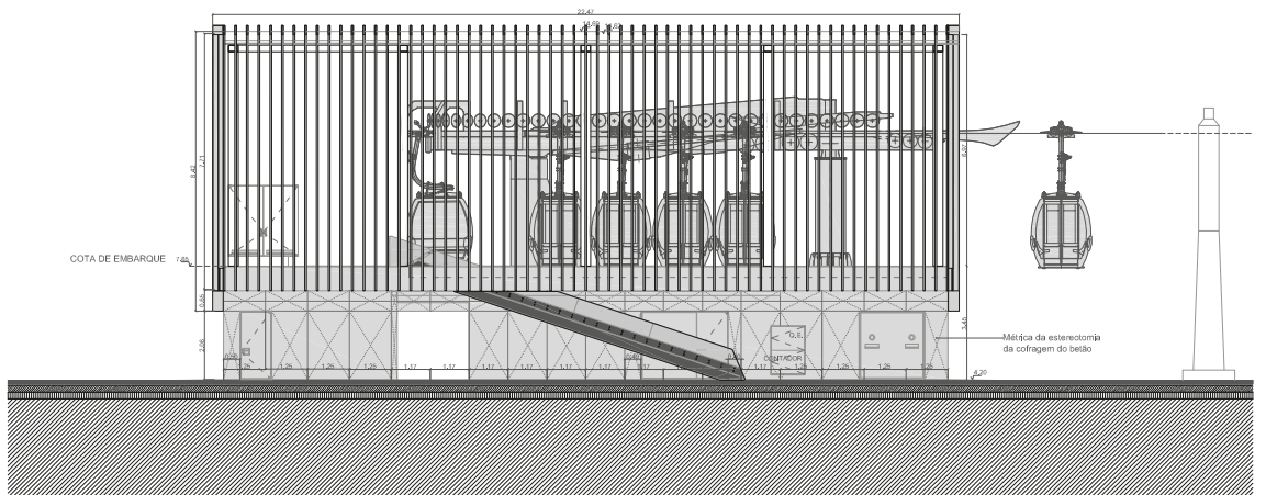
alçado sul
