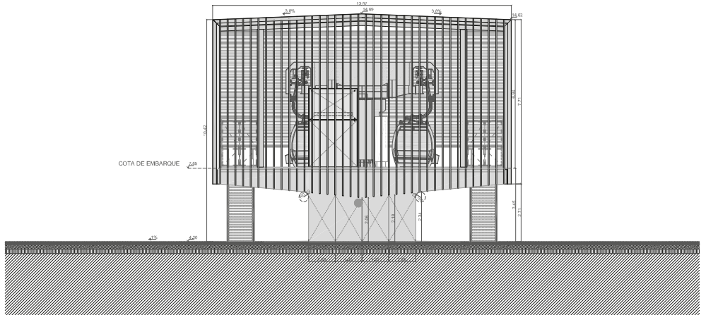
alçado poente
