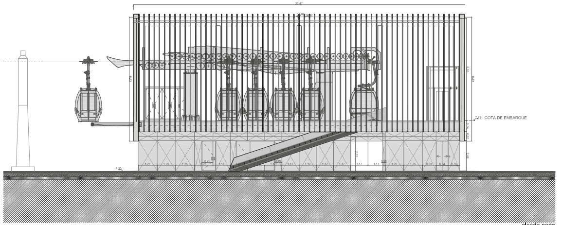
alçado norte
