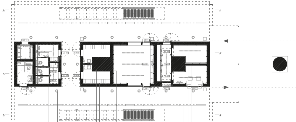
planta piso 1
